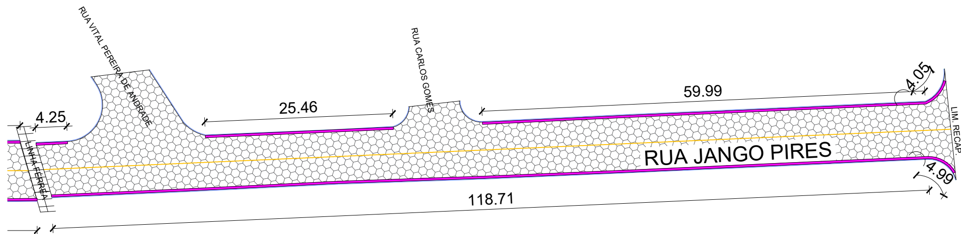
PLANTA BAIXA DE LOCAÇÃO DAS SARJETAS ESCALA 1:1.000
