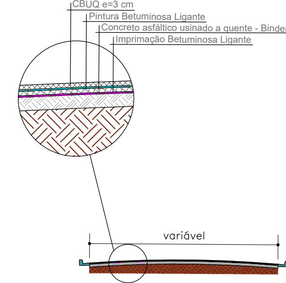
PERFIL TRANSVERSAL GERAL SEM ESCALA
