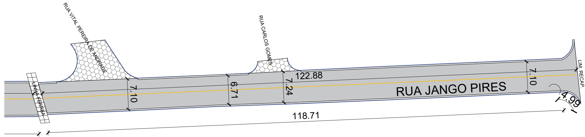
PLANTA BAIXA DE ÁREA DE RECAPEAMENTO ESCALA 1:1.000
